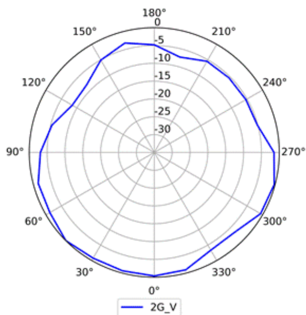
2.4GHz (垂直)
