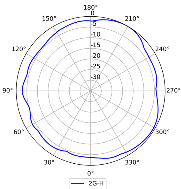
2.4GHz (水平)
