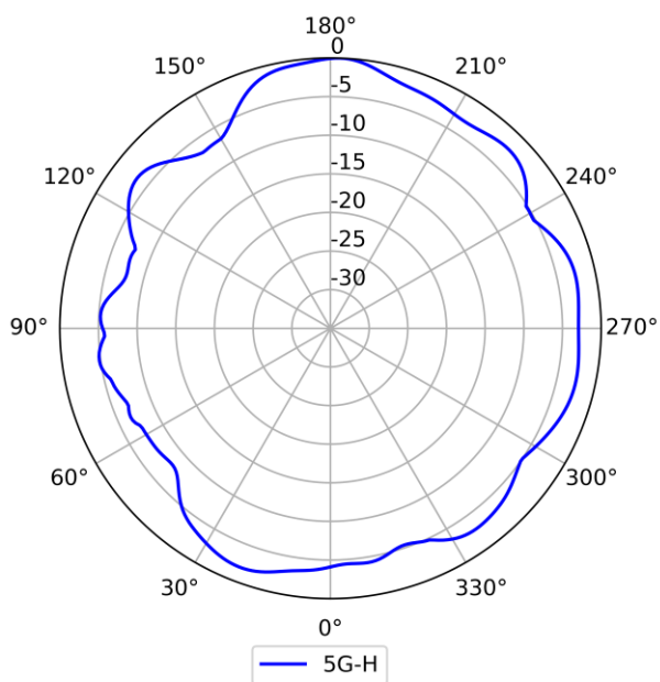
5GHz (水平)
