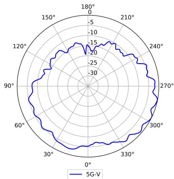
5GHz (垂直)
