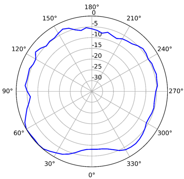
5GHz (水平)
