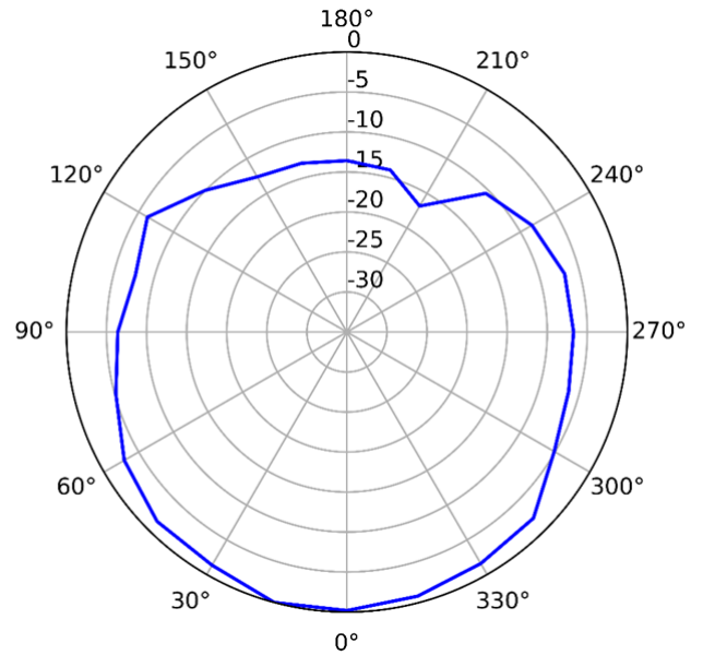
5GHz (垂直)
