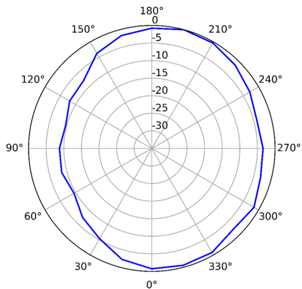
2.4GHz (垂直)
