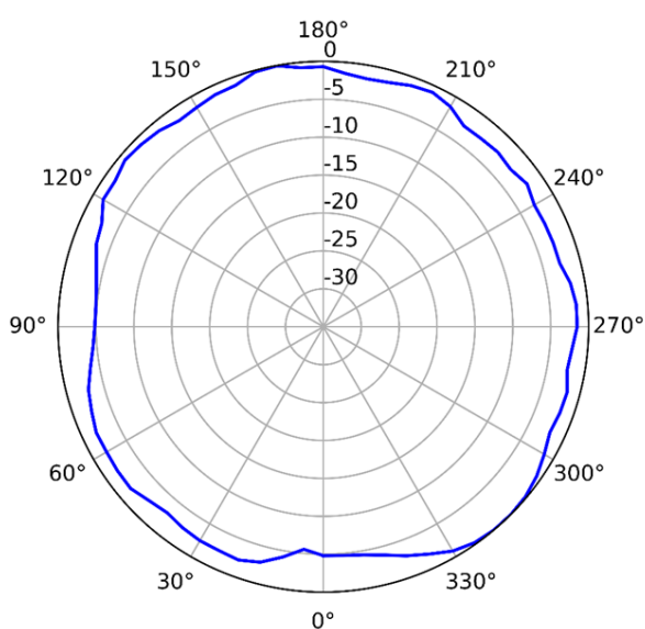
5GHz (水平)
