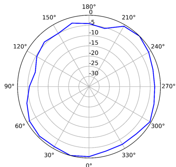
5GHz (垂直)
