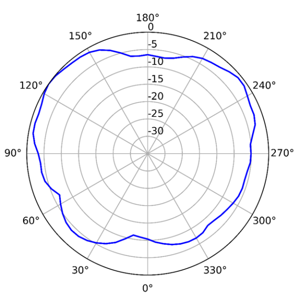
2.4GHz (水平)
