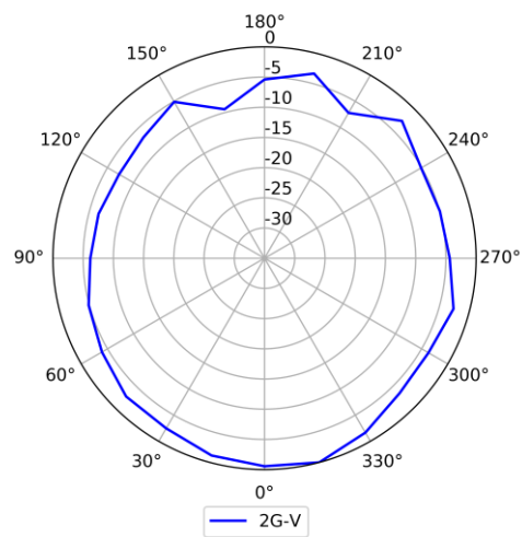
2.4GHz (垂直)
