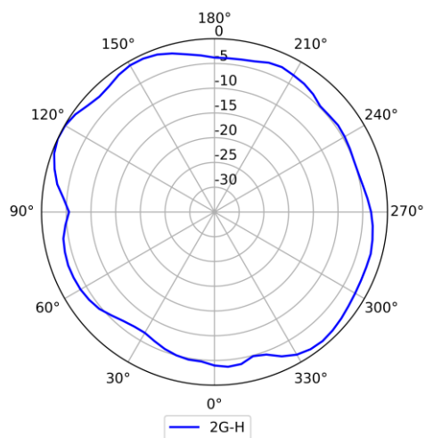
2.4GHz (水平)
