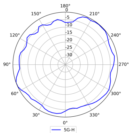
5GHz (水平)
