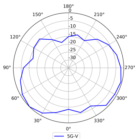
5GHz (垂直)
