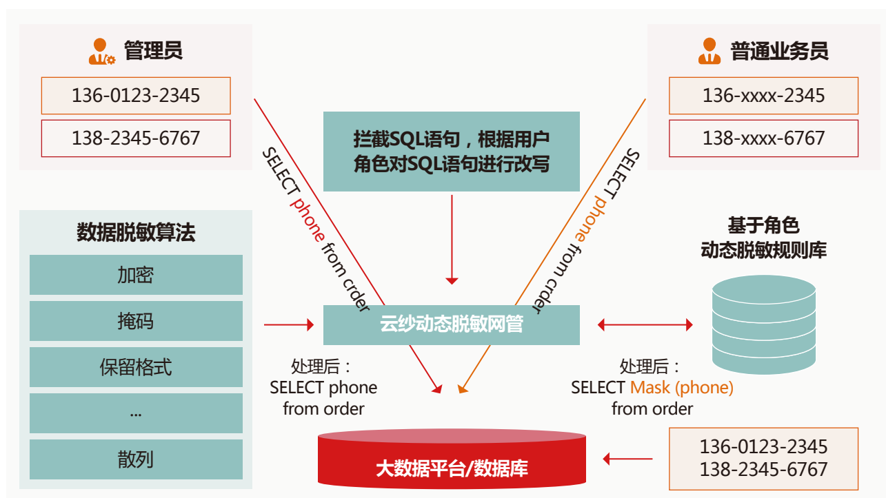
图 65 自适应脱敏算法
