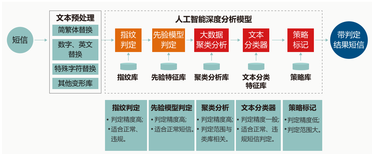
图 62 基于人工智能的垃圾短信综合判定模型
