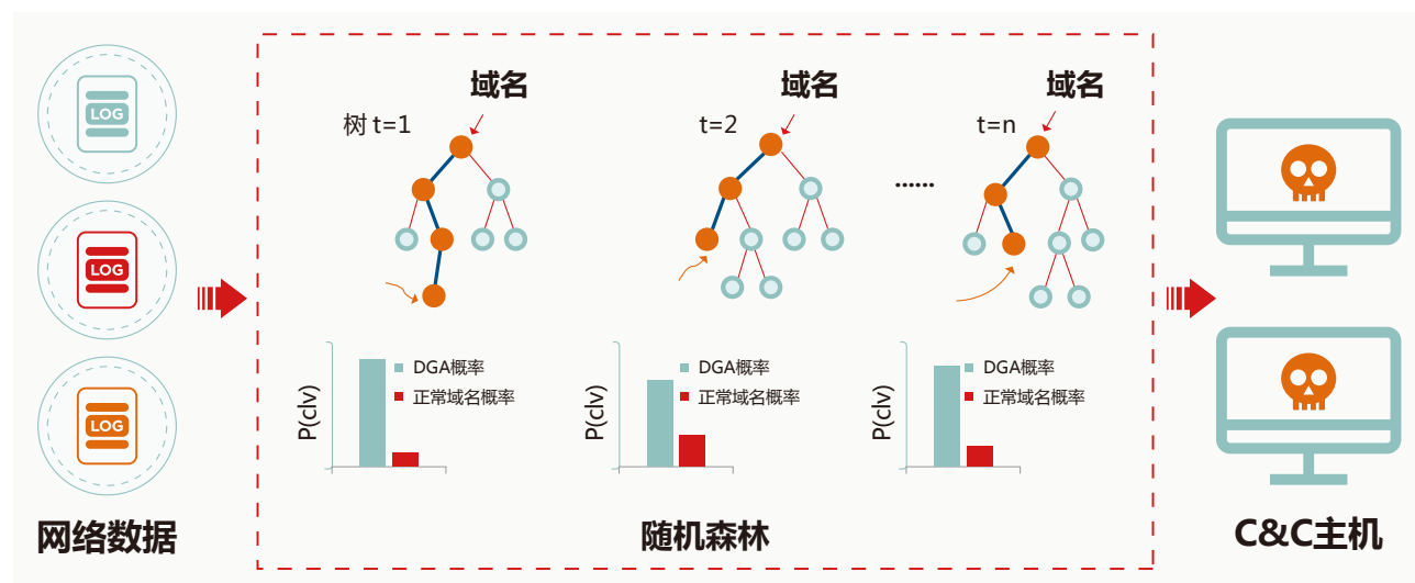
图 67 基于人工智能的僵尸网络C&C服务器检测工作流程图
